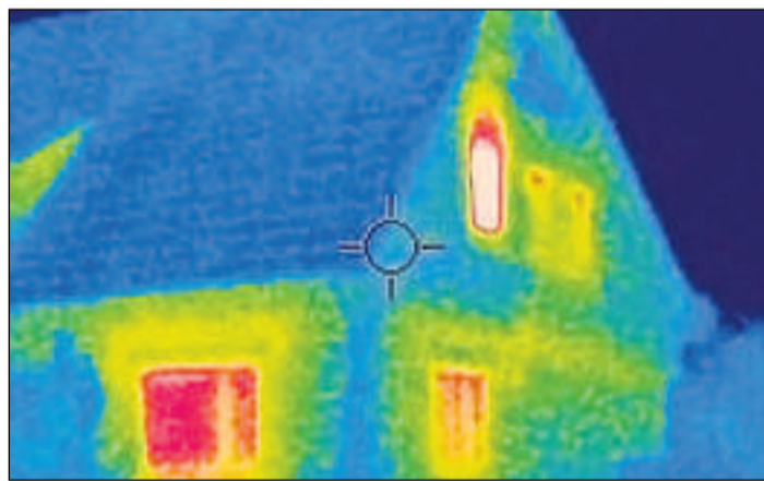
Vorher: Die roten Flächen (Bild oben) zeigen, wo die Wärme aus dem Haus entweicht. Nachher: Rote Flächen sind nur noch in geringem Maße zu erkennen. Die Modernisierung hatte Erfolg.
